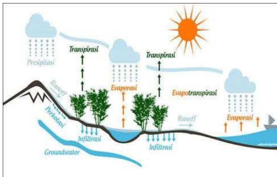
Gambar 3.3 : Siklus Hidrologi (Asdak, 2010)
