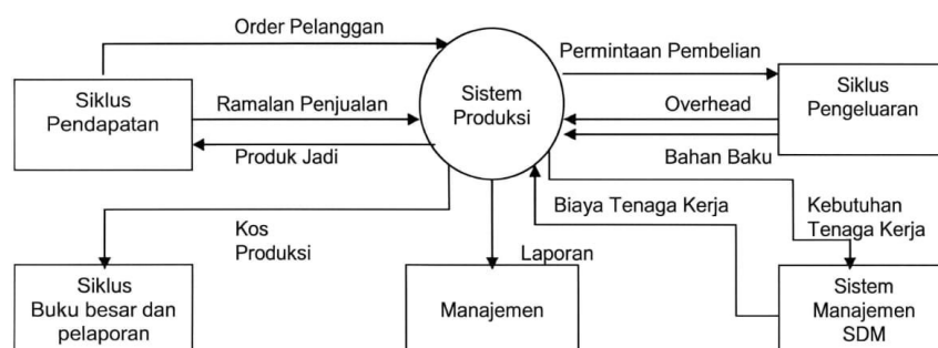
Gambar 2.3 Siklus Produksi
