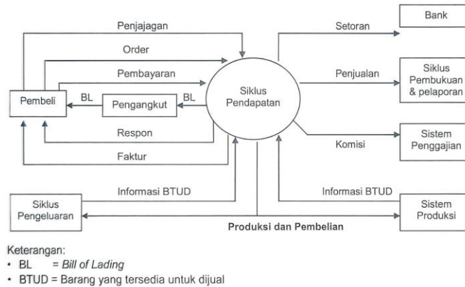
Gambar 2.1 Siklus Pendapatan
