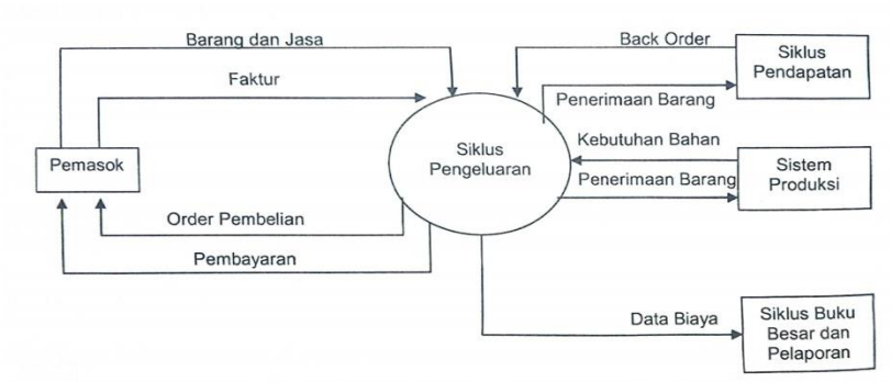
Gambar 2.2 Siklus Pengeluaran
