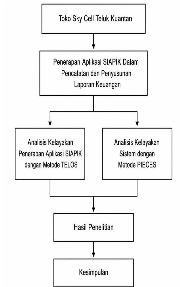
Gambar 2.13 Kerangka Pemikiran
